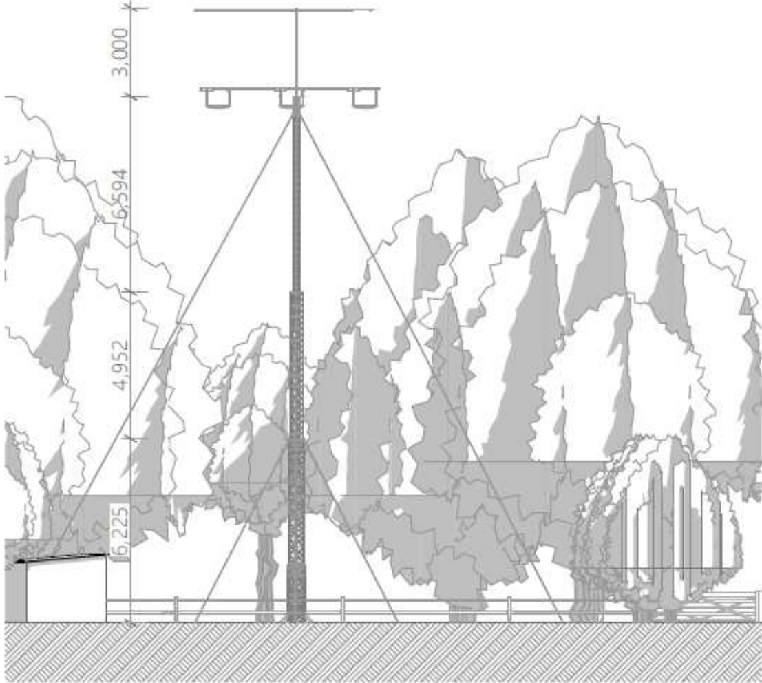
E1 South 1:100
