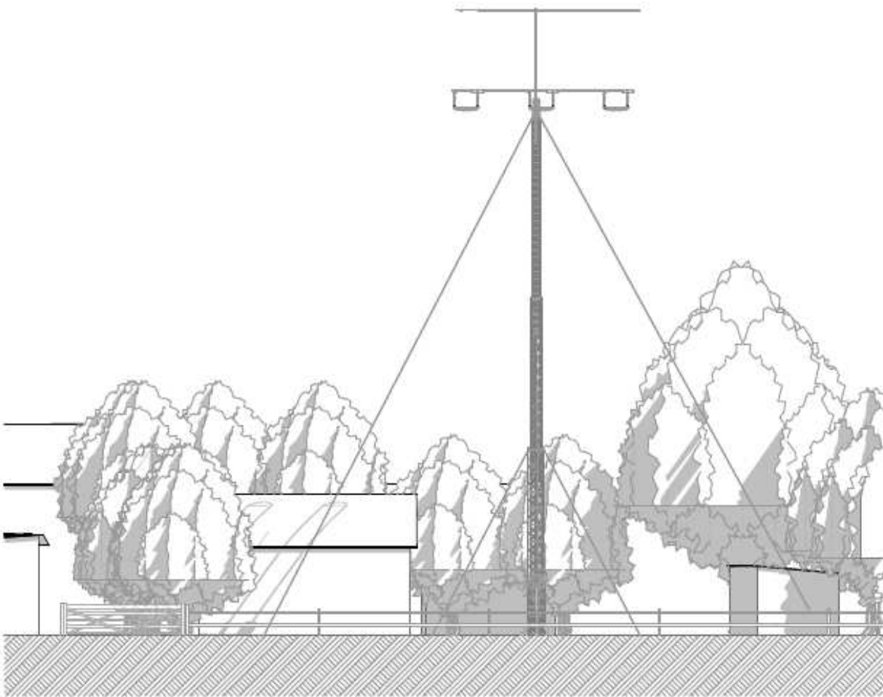
E3 North 1:100
